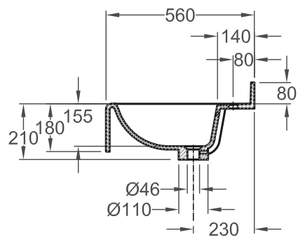
VARICOR Preciosa Pro Comfort Waschtisch-Schnitt 30.04.2004/Re
