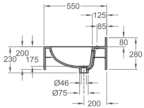
VARICOR Wetsset Plus Waschtisch-Schnitt 19.10.2011/Re-Th
